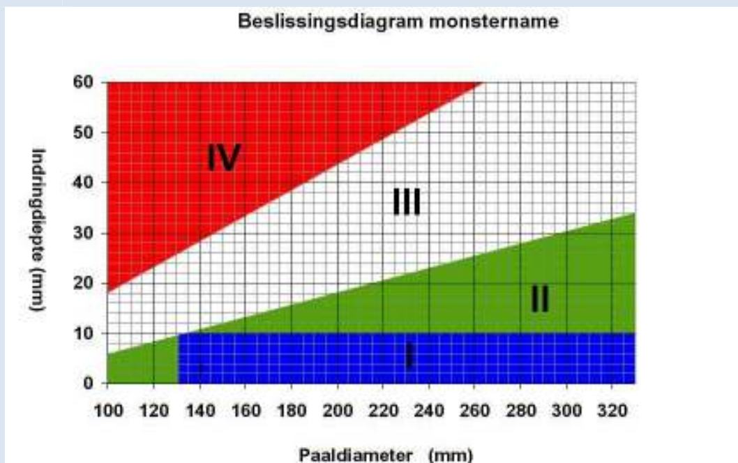
Grafiek 2.1. Beslissingsdiagram voor het nemen van monster, welke gebaseerd is op normaal voorkomende situaties met betrekking tot de verhouding paaldiameter en belasting (100 mm en 30 kN; 150 mm en 60 kN; 200 mm - grotere diameters en 150 kN).
